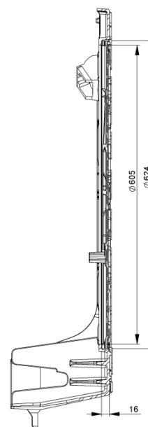
A-A (1:5)
