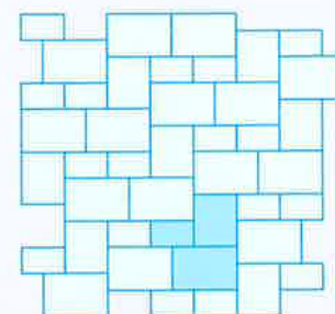
Pose type „Allgäu 1“ 26,25 x 17,5/17,5 x 10,5/21 x 17,5
