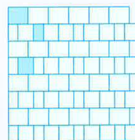
Pose alternée 21 x 17,5/17,5 x 10,5/17,5 x 15,75
