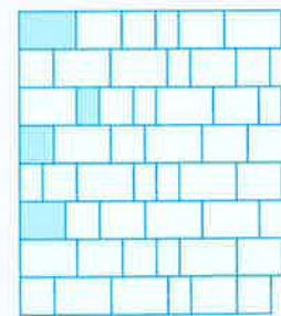
Pose alternée 26,25 x 17,5/17,5 x 15,75/ 21 x 17,5/17,5 x 10,5
